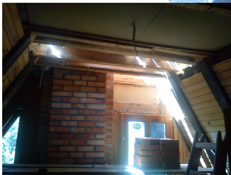
Przebudowa kominia z nowym metalowym wkładem
