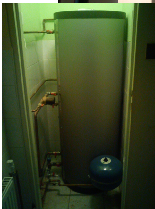
Nowy 200 l. zbiornik na podgrzewaną przez kominę wodę, zamontowany w pomieszczeniu toalety.
